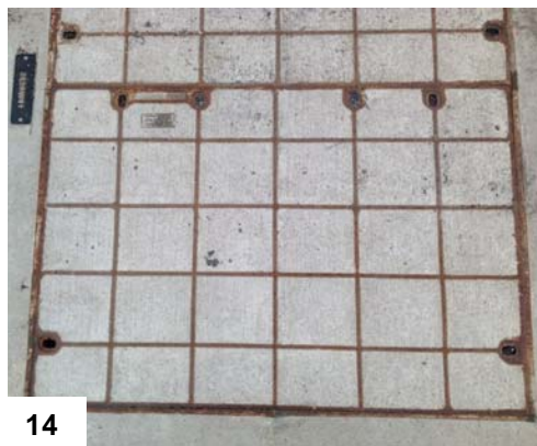
abhängig vom Deckelgewicht/ Deckelgröße mit einem oder zwei KänguruLifter® Tandem und Krafthaken-T
